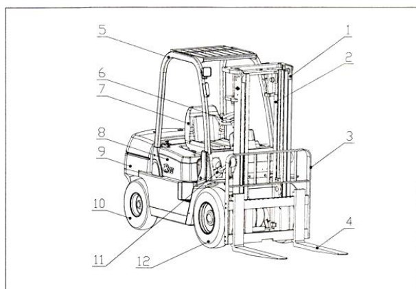
Rys. 1. Wózek widłowy: 1 – maszt, 2 – siłownik, 3 – krata ochronna, 4 – widły, 5 – rama bezpieczeństwa, 6 – kierownica, 7 – fotel, 8 – pokrywa silnika, 9 – przeciwwaga, 10 – koło tylne, 11 – siłowniki przechyłu, 12 – koło przednie [9]
