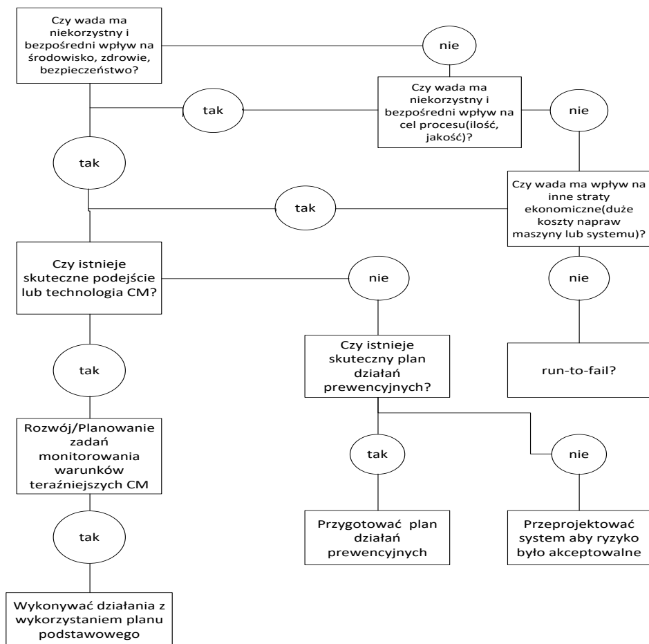
Rys. 7. Diagram drzewa logicznego dla RCM [1]
